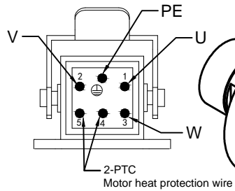
【Wiring description diagram】
