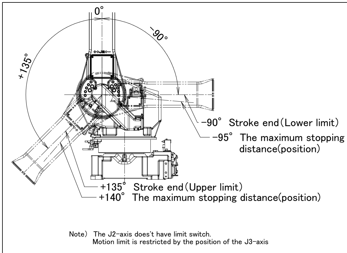
Fig. 3.3 (d) J2-axis motion limit (M-710iC/50/70/50H/45M/50E)
