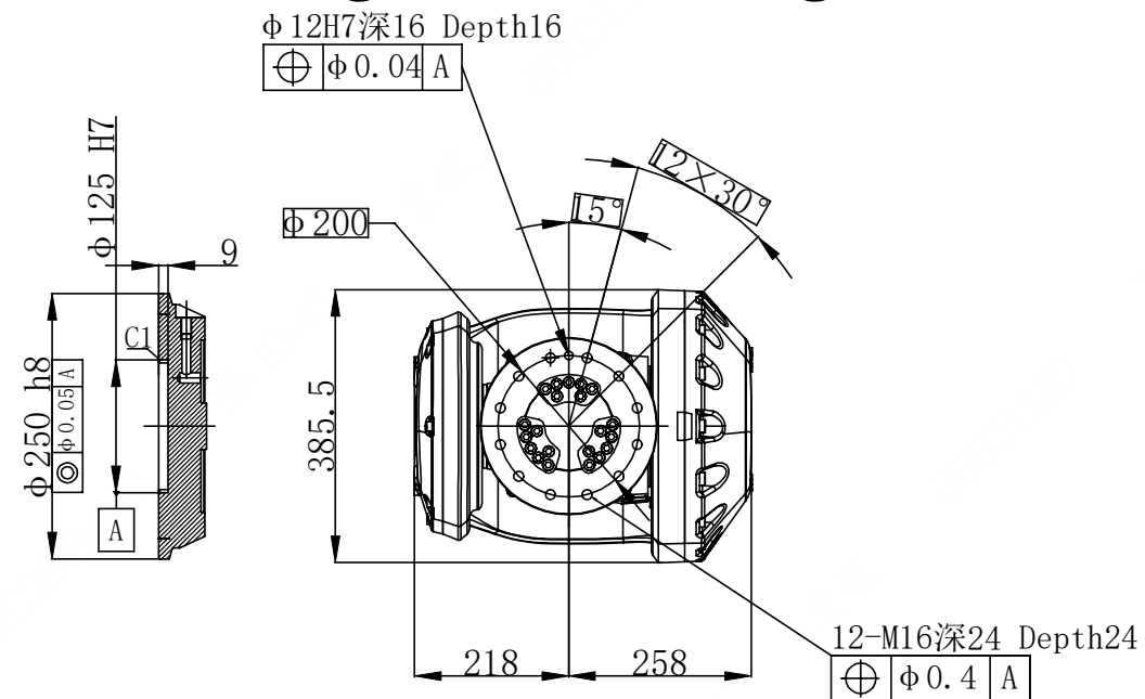
末端法兰安装图 (End flange mounting size)
