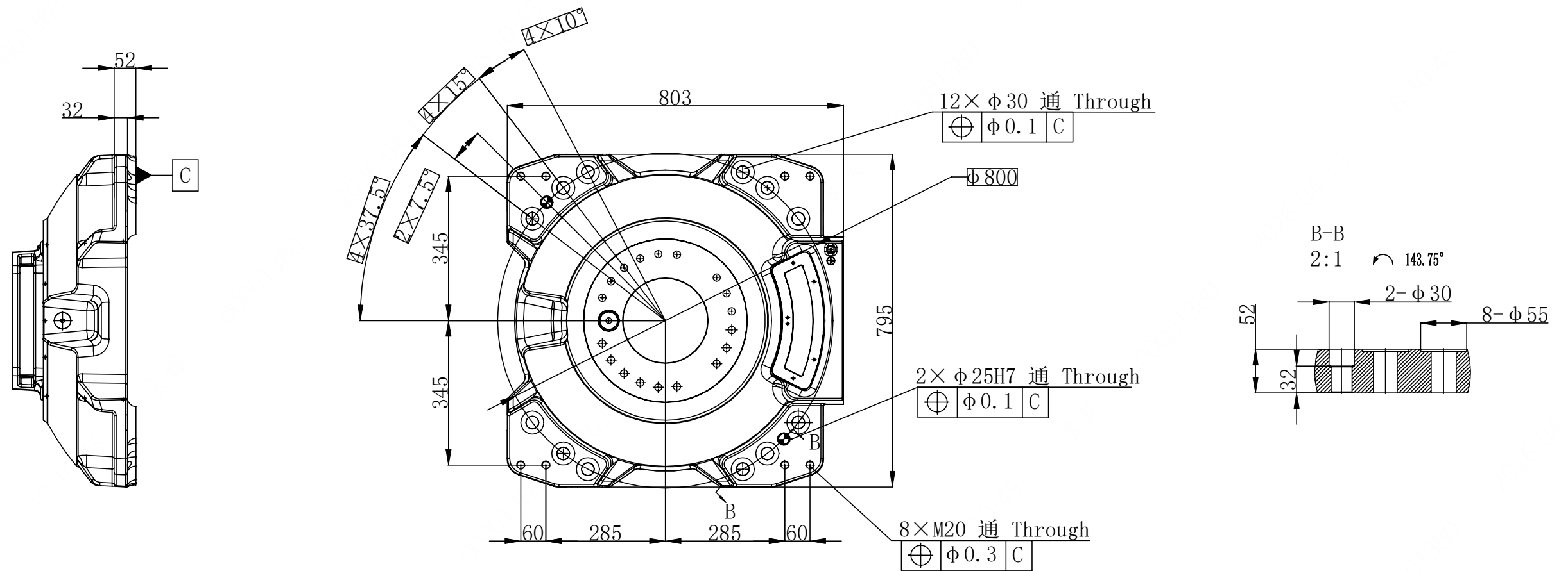
末端法兰安装图 (End flange mounting size)
